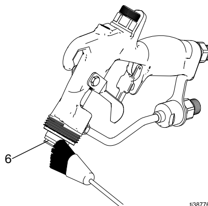
FIG. 38: Limpiar el exterior del difusor
