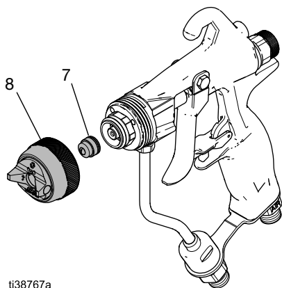
FIG. 26: Retirar el conjunto del cabezal de aire y la boquilla de pulverización
