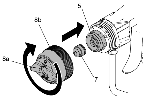
FIG. 40: Volver a montar la boquilla de pulverización y el cabezal de aire
