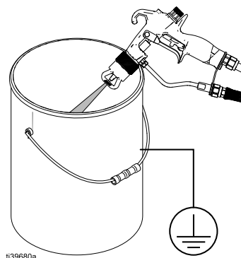
FIG. 27: Limpiar la pistola
