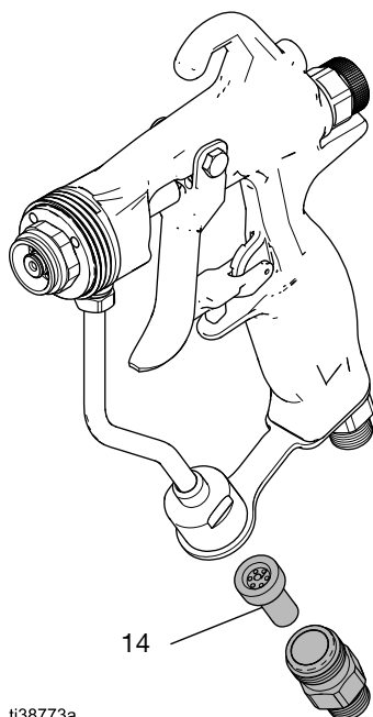
FIG. 31: Revise el filtro de fluido en línea
