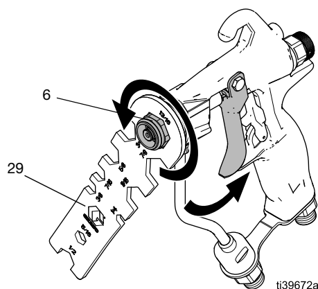
FIG. 50: Quitar el cartucho de fluido
