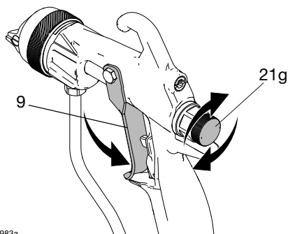
FIG. 32: Revise el gatillo y la perilla de ajuste del abanico
