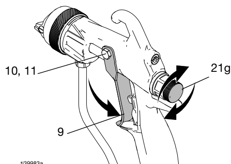
FIG. 41: Revisar el gatillo y la perilla de ajuste del abanico
