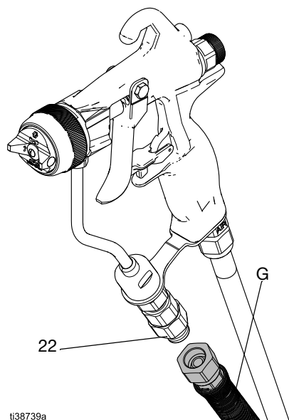
FIG. 6: Conexión de la manguera de suministro de fluido a la pistola
