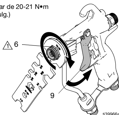
FIG. 52: Presionar el gatillo mientras enrosca el cartucho
