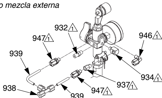
FIG. 37: Detalles de la bomba de catalizador
