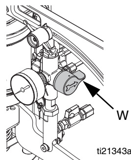
FIG. 9: Válvula de alivio de presión de la bomba de catalizador
