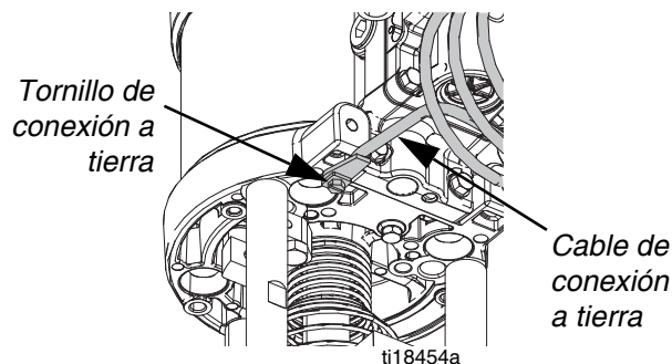
FIG. 5: Cable de conexión a tierra
