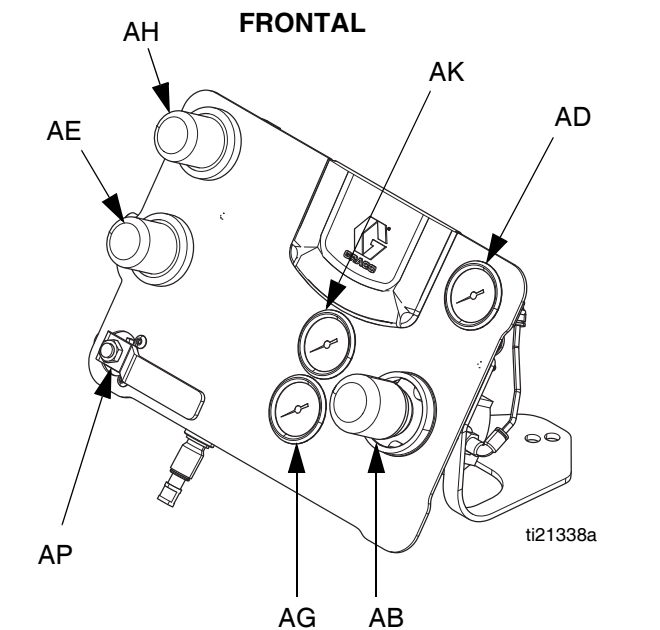
Fig. 7: Componentes del tablero de control de aire
